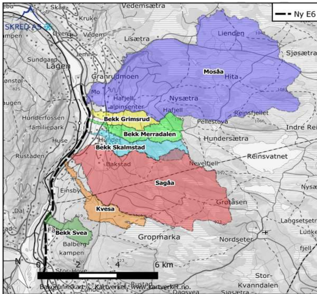
Figur 4-10 Identifiserte feltgrenser for de berørte vassdragene (Kilde E6 Storhove - Øyer Hydrologirapport, Skred AS)
