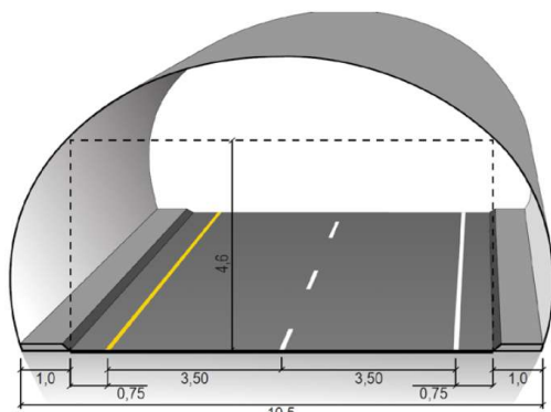
Figur 4-4 Normalprofil for tunnel T10,5 (fra SVV håndbok N100). Avstand mellom tunneløpene vil være ca. 10 m
