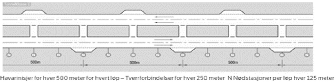
Figur 4-5 Tunnelklasse E, havarinisjer, nødstasjoner og tverrforbindelser (fra SVV håndbok N100)
