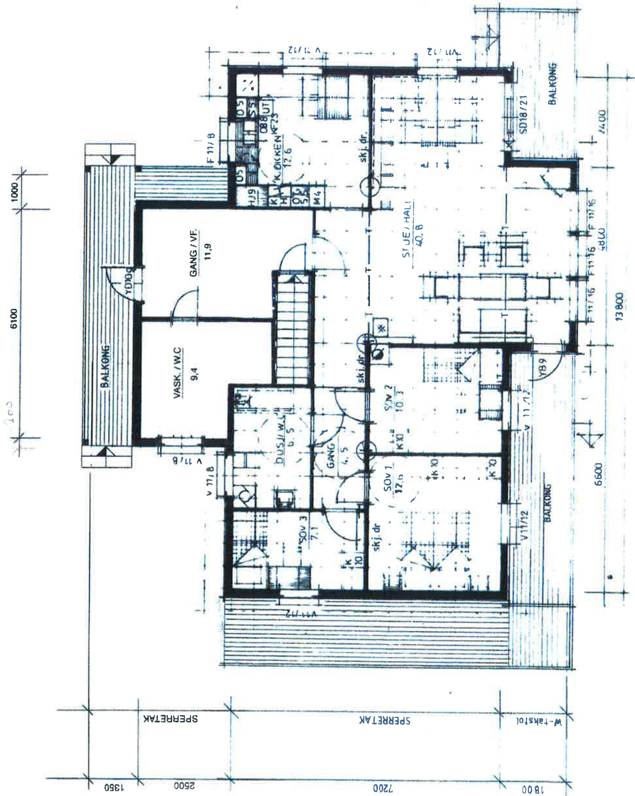
PLAN 1. ETG.
