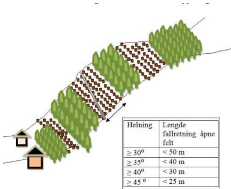
Figur 2: Skisse av hogstfelt med redusert lengde på fallretning med åpne arealer. Dette for å hindre utløsning av snøskred med betydelig skadepotensiale. Tabell for største lengde i fallretning er for snøskred (NGI, 2015).
