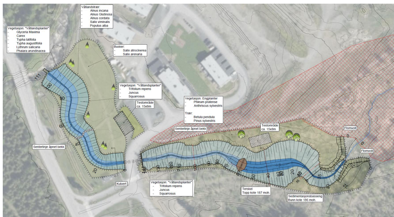
Figur 1. Skisse av planlagt tiltak ifb. med åpning av Trodalsbekken.
